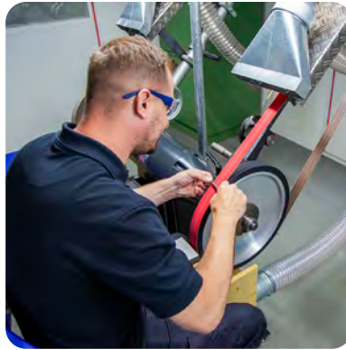
Schleifen der Titanteile
