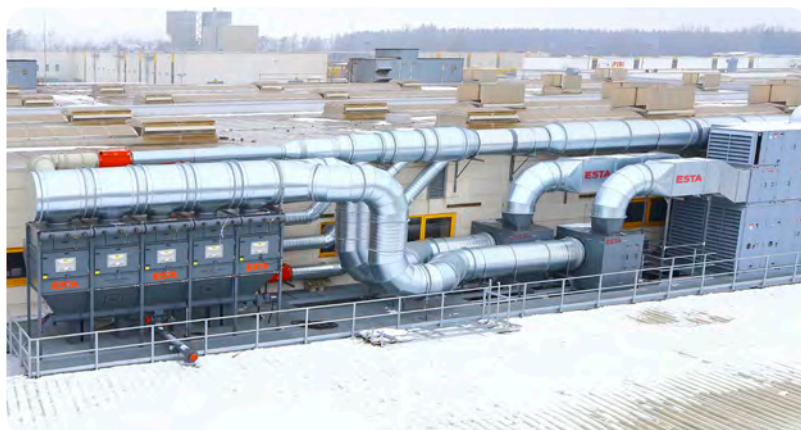
Absaugsystem ist auf dem Dach der Produktionshalle installiert
