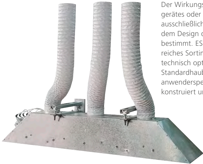
Absaughaube mit Drucklufteinblasung
