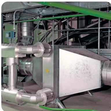
Rohrleitungssystem für Abluft mit integriertem Kühler
