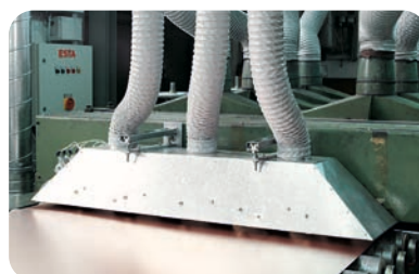
Spezialhaube 120 x 30 cm
