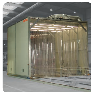
Fahrbare Absaugkabine für die Rotorblattfertigung
